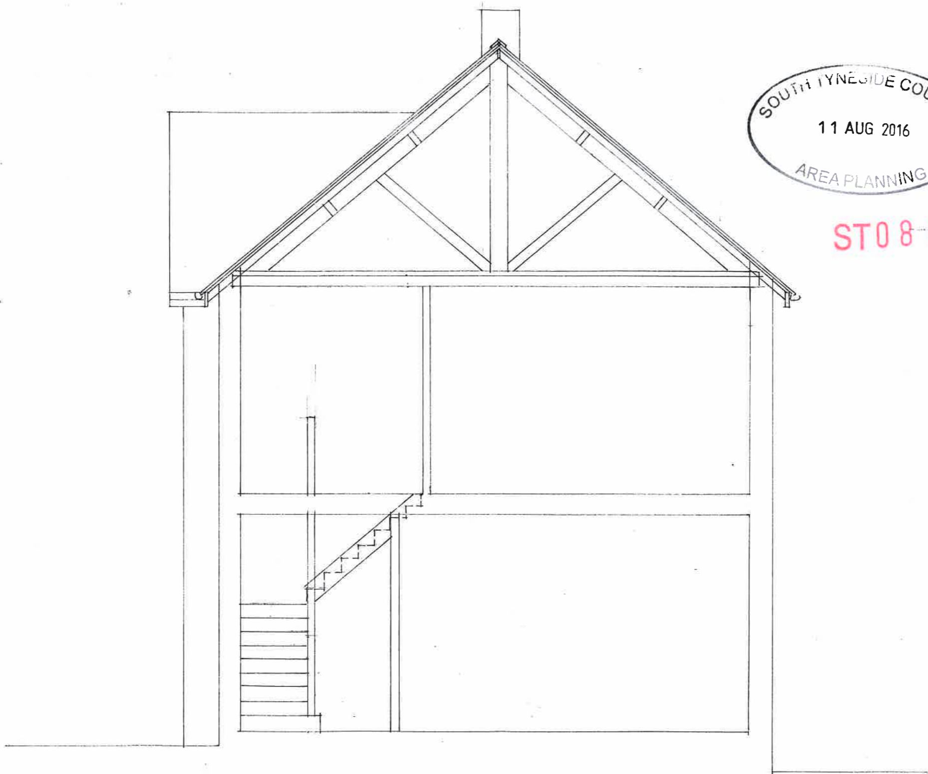
SECTION A-A
